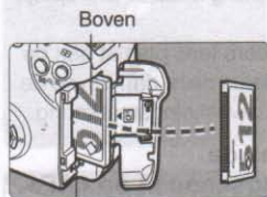
CF-kaart uitwerpknop
